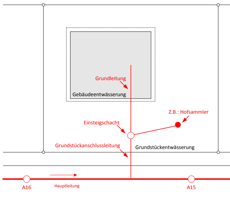
Abbildung 1: Liegenschaftsentwässerung
