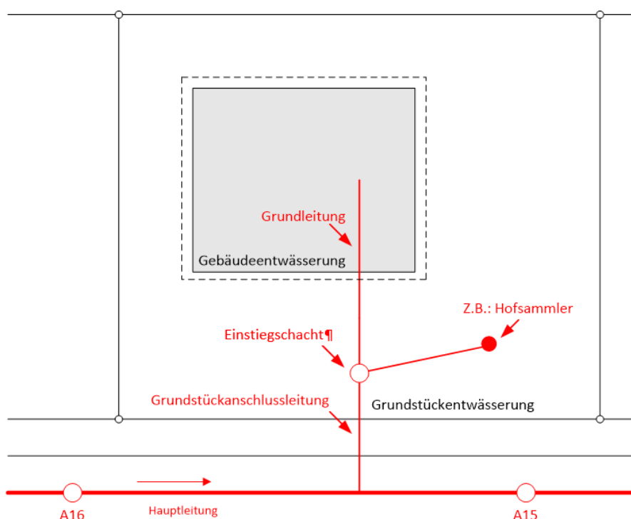
Abbildung 1: Liegenschaftsentwässerung
