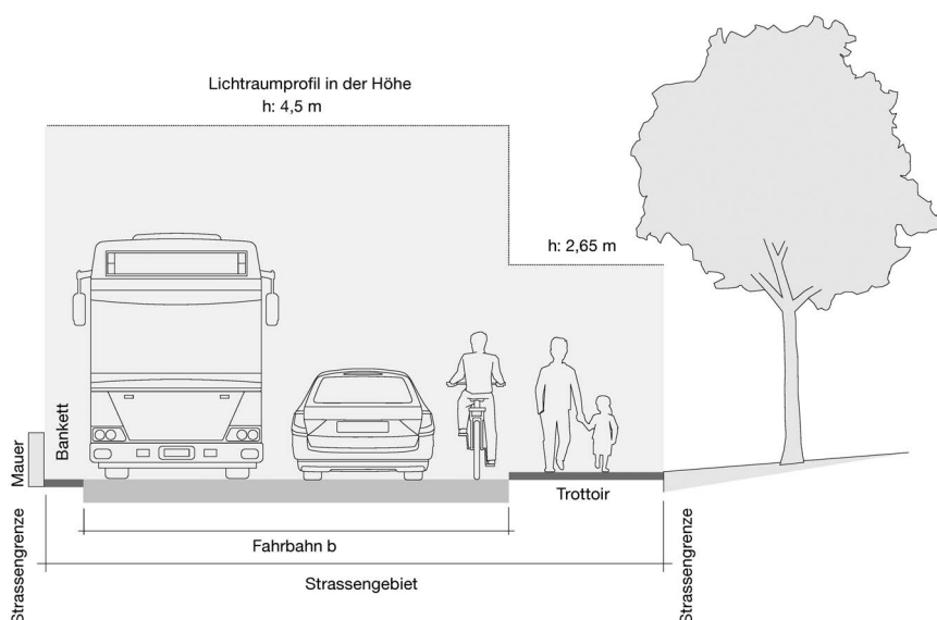
Abbildung: Frei zu haltender Lichtraum gemäss Anhang 5 der Verordnung in Ergänzung zu den Abständen (§ 27 b)
